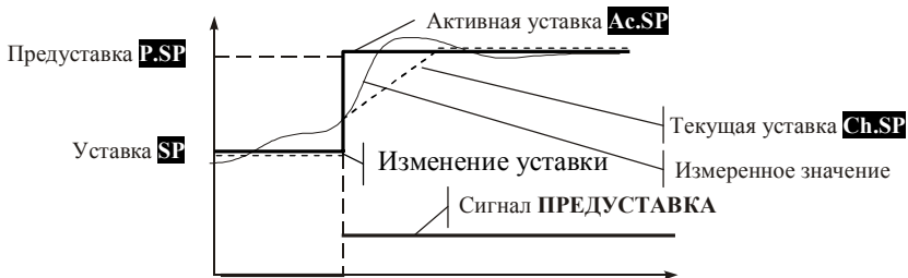
Рисунок 5.3 – Уставки регулятора
