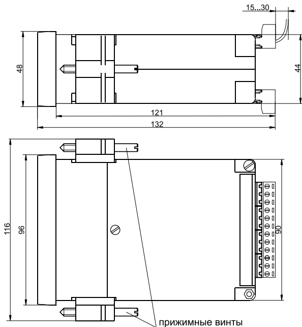
Рисунок 6.1 – Габаритные размеры прибора МЕТАКОН-6305
