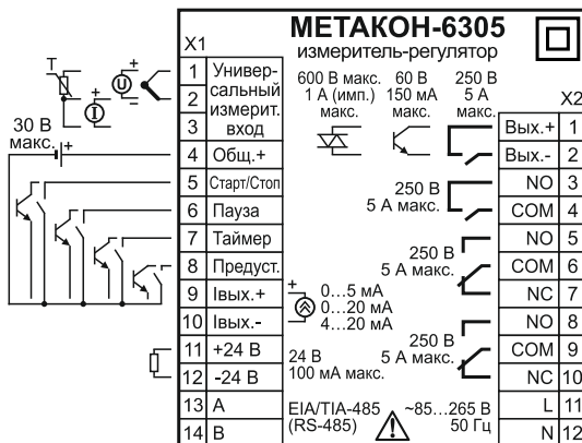
Рисунок 6.2 – Электрическая схема подключения прибора МЕТАКОН-6305
