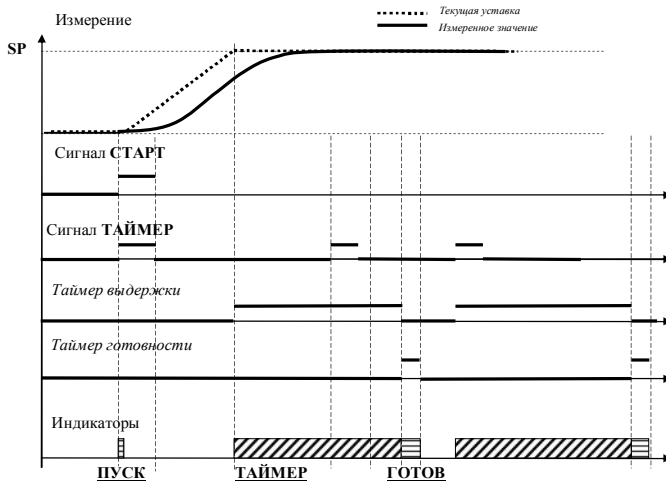
Рисунок 5.13 – Диаграмма работы таймера выдержки с условным запуском сигналом ТАЙМЕР по уровню текущей уставки
